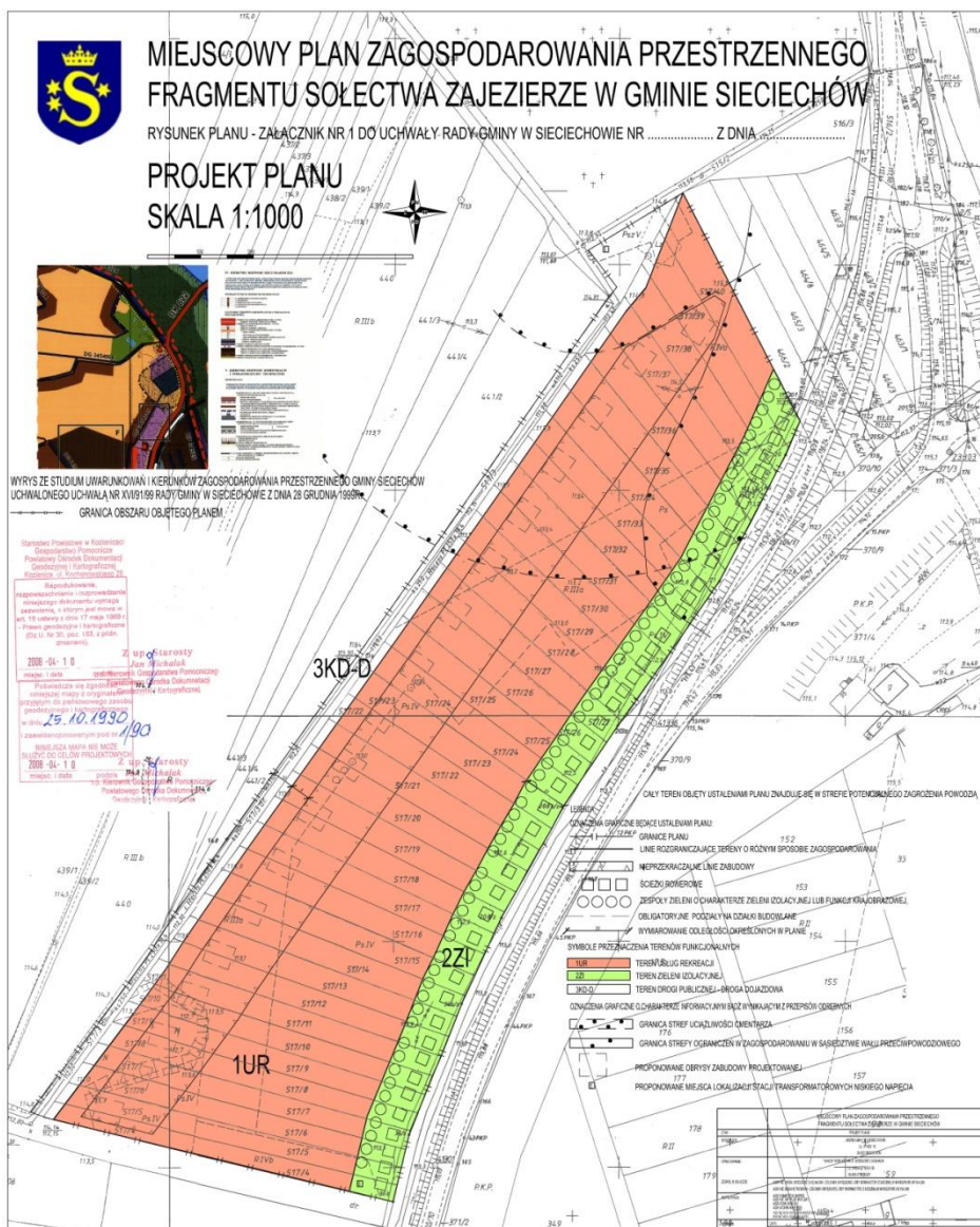
Miejscowy plan zagospodarowania przestrzennego fragmentu sołectwa Zajezerze
