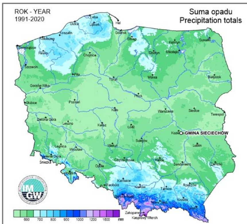
Rysunek 5. Mapy klimatu Polski z zaznaczoną przybliżoną lokalizacją gminy Sieciechów – suma opadów w latach 1991-2020
