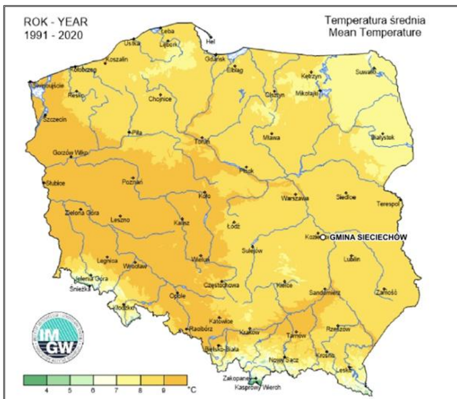
Rysunek 3. Mapa klimatu Polski z zaznaczoną przybliżoną lokalizacją gminy Sieciechów – średnia temperatura w latach 1991-2020
