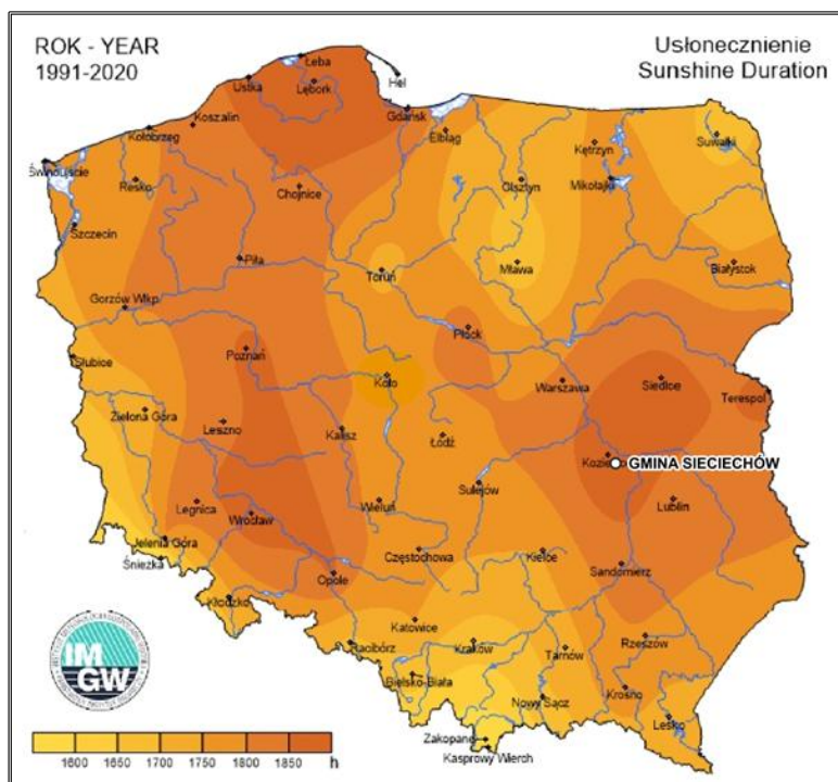
Rysunek 6. Mapy klimatu Polski z zaznaczoną przybliżoną lokalizacją gminy Sieciechów – usłonecznienie w latach 1991-2020
