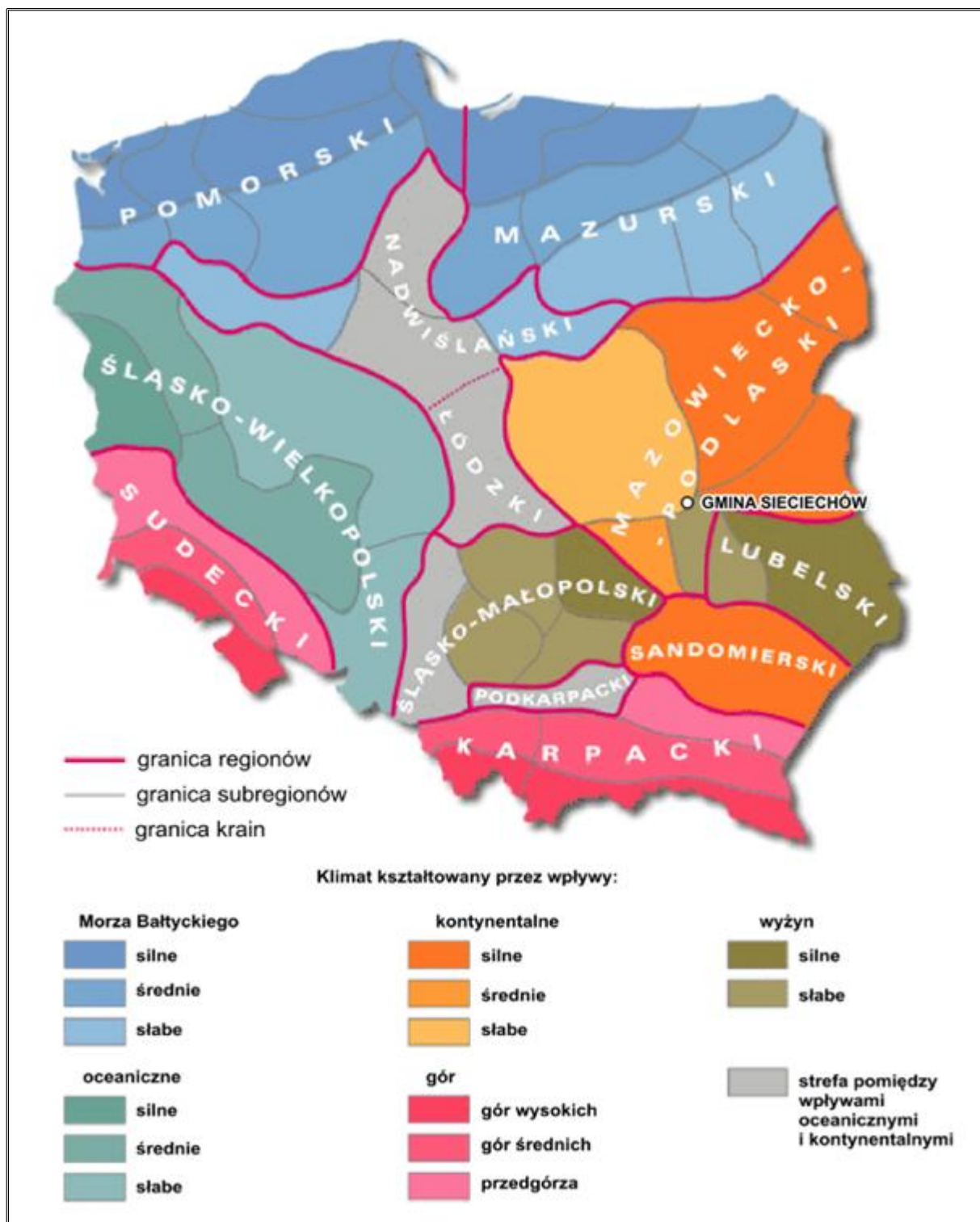
Rysunek 2. Mapa podziału Polski na regiony klimatyczne W. Okołowicza, D. Martyn z zaznaczoną lokalizacją gminy Sieciechów
