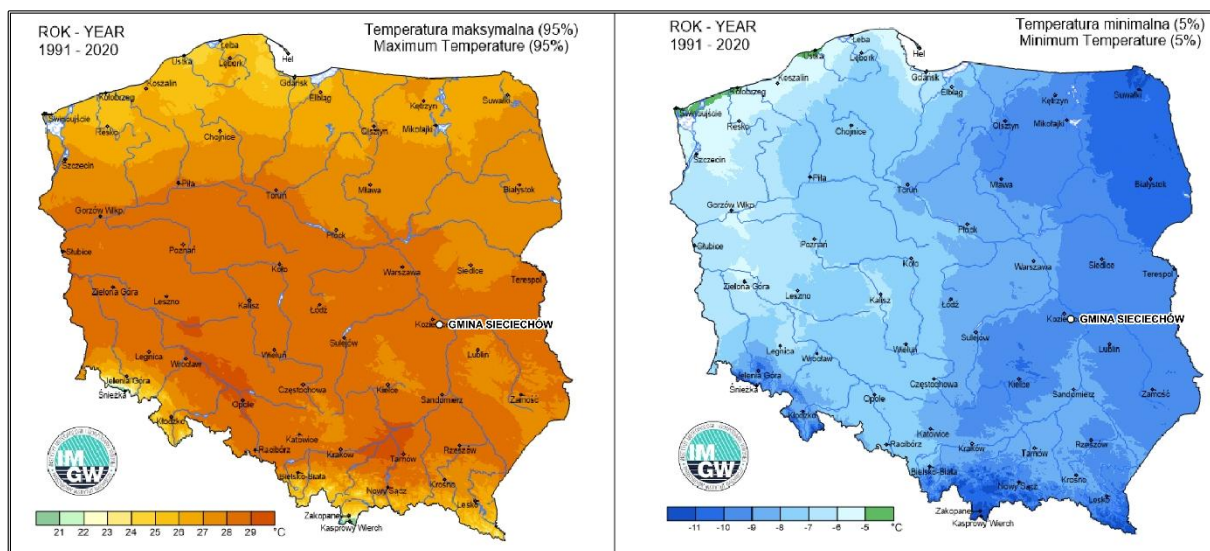
Rysunek 4. Mapa klimatu Polski z zaznaczoną przybliżoną lokalizacją gminy Sieciechów – temperatura maksymalna i temperatura minimalna w latach 1991-2020
